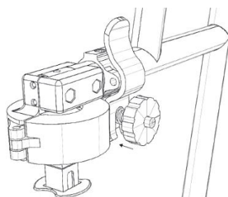
Durch Anziehen des Handgriffes wird die Feder des Bremsmechanismus zusammengedrückt.
